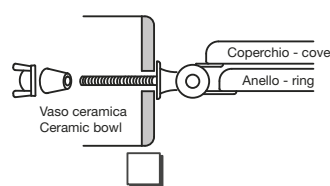
Cerniere per vaso con fori orizzontali Hinges for vase with horizontal holes
