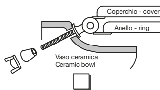
Cerniere per vaso con fori obliqui Hinges for vase with oblique holes
