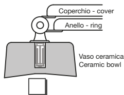
Cerniere per vaso con fori ciechi Hinges for pots with blind holes
